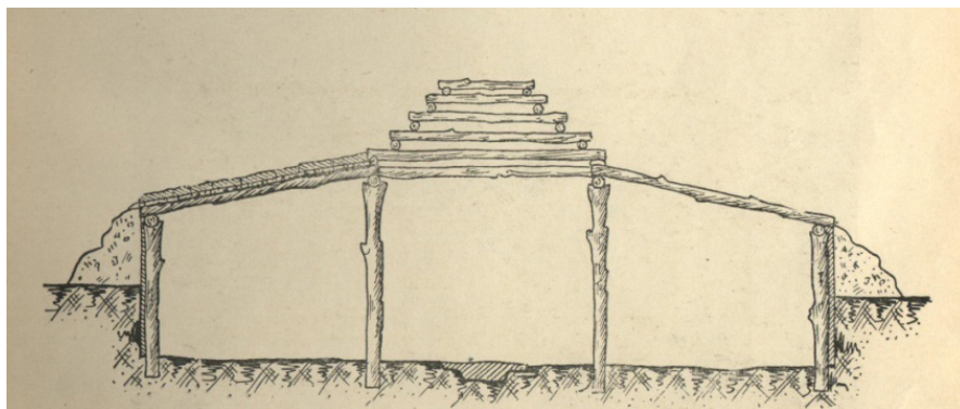
3-сурет. Қола дәуіріндегі үй төбесін жиде, қарағашпен жабу әдісі. Сызба «Марғұлан Ә., Бәсенов Т., Меңдіқұлов М. Қазақстан архитектурасы» (Алматы: Қазақ Мемлекет баспасы, 1959) атты еңбектен алынды
